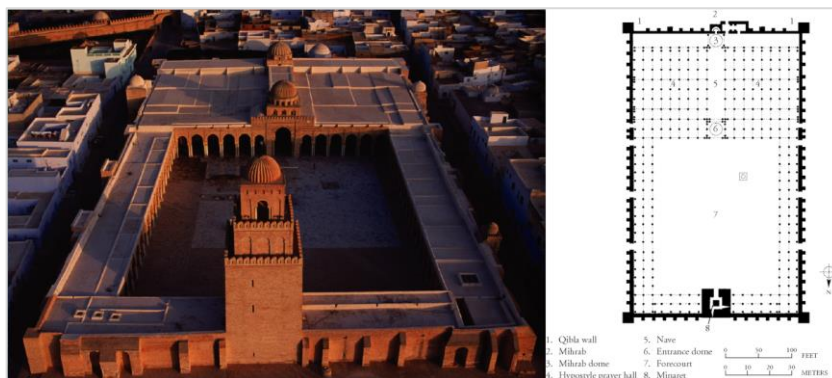
Gambar 4. Tipe Masjid Hypostyle Hall di daratan Arabia, Spanyol dan Afrika Utara
